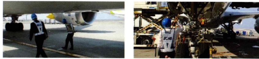
機体の胴体・主翼(エンジン含む)・脚などに部品欠落・着氷等がないか点検
