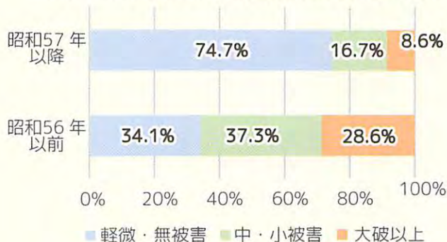
阪神・淡路大震災における建築時期による被害状況
